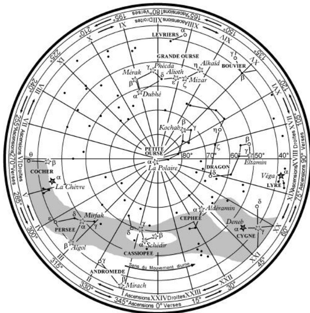
Carte de l'hémisphère céleste Nord pour les déclinaisons de 35° N à 90° N
